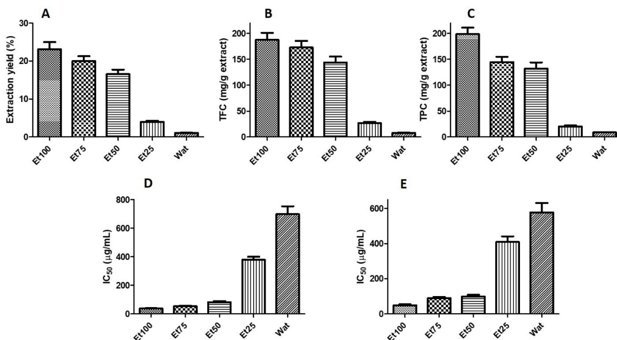
Gambar 1. Hasil ekstraksi (A), TKFl (B), TKFe (C), nilai IC 50 terhadap DPPD (D) dan nilai IC 50 terhadap peroksidasi lipid (E) ekstrak kasumba turate yang diperoleh dari pelarut yang berbeda (mean \pm SD, n=3 )
