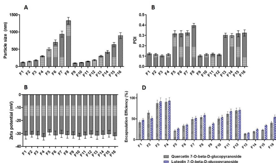
Gambar 3. Hasil ukuran partikel (A), PDI (B), potensial zeta (C) dan enkapsulasi untuk NLP yang dibuat dari ekstrak kasumba terate (rata-rata \pm SD, n=3 )
