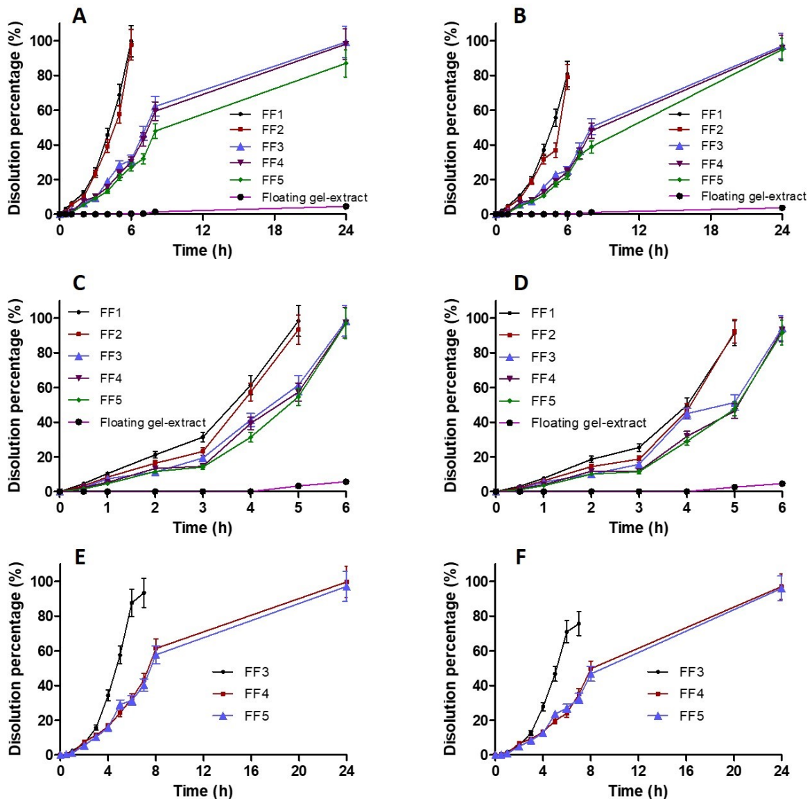
Gambar 8. Profil disolusi in vitro quercetin 7-O-beta-D-glucopyranoside (A) dan luteolin 7-O-beta-D-glucopyranoside (B) dari NLP-dry floating gel in situ pada FaSSGF, Profil disolusi in vitro quercetin 7-O-beta-D-glucopyranoside (C) dan luteolin 7-O-beta-D-glucopyranoside (D) dari NLP-dry floating gel in situ pada FaSSGF, Profil disolusi in vitro quercetin 7-O-beta-D-glucopyranoside (E) dan luteolin 7-O-beta-D-glucopyranoside (F) dari NLP-dry floating gel in situ pada FaSSGF setelah berada 2 jam pada FaSSGF (rata-rata \pm SD, n=3)
