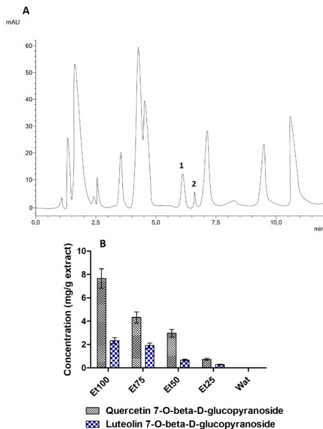
Gambar 2. Kromatogram HPLC quercetin 7-O-beta-D-glucopyranoside (1) dan luteolin 7-O-beta-D-glucopyranoside (2) dalam ekstrak kasumba turate (A). Konsentrasi kedua senyawa ekstrak kasumba turate diperoleh dari pelarut yang berbeda (B) (mean \pm SD, n=3)
