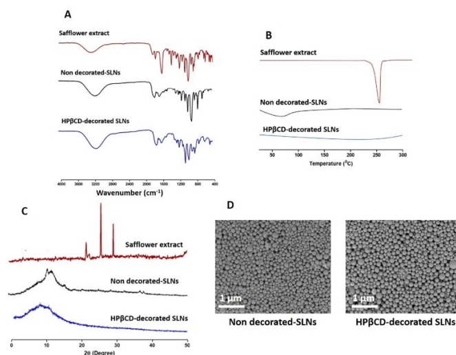
Gambar 4. Hasil evaluasi FTIR (A), DSC (B), XRD (C) dan SEM (D)
